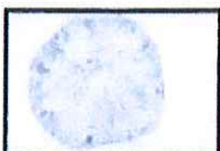
Chloroform
